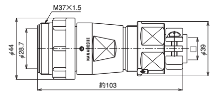
NJW-323C・324C-AdM (正芯) NJW-323C・324C-AdF (逆芯)
