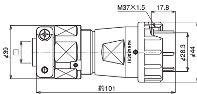
NJW-323C・324C-PF (正芯) NJW-323C・324C-PM (逆芯)
