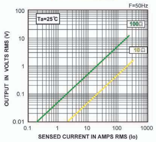
CT2000
