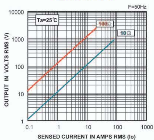
JCTP-80 / JCTH-80
