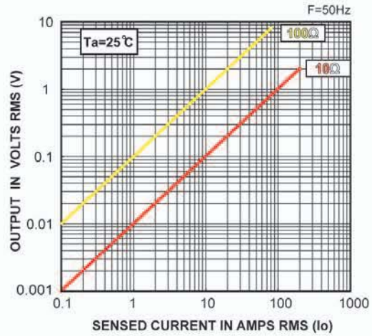
JS51V / JS51W
