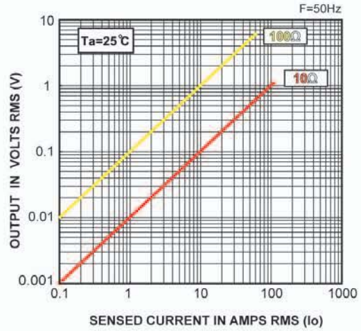
JS41V / JS41W
