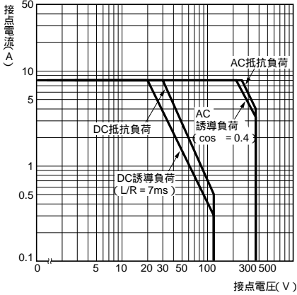
形G2R-14、形G2R-1A4
