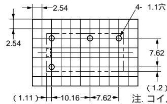
プリント基板加工寸法 (BOTTOM VIEW) 寸法公差は±0.1mmです。
