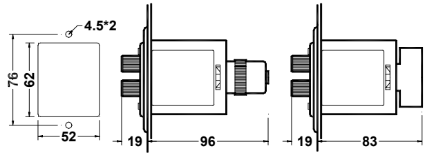
INSERT HOLE STDV- Y + US-08。 STDV- Y + P3G-08
