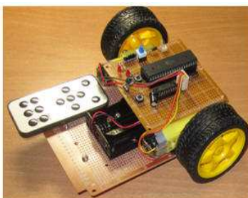
紅外線遙控車 CARC
