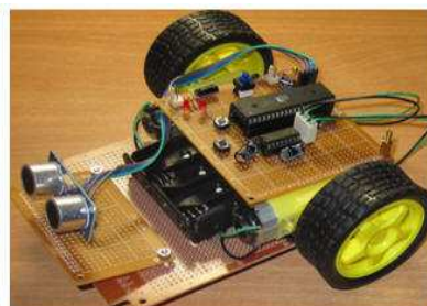
超音波避障車 CASO
