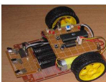
紅外線避障車 CARL
