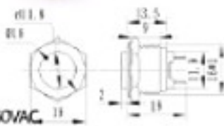
S16023A 16mm不鏽鋼金屬平面中心燈無段開關(焊線式)
