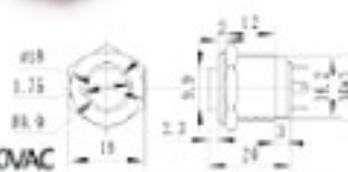
S16002A 16mm不鏽鋼金屬平面無段開關(單刀)
