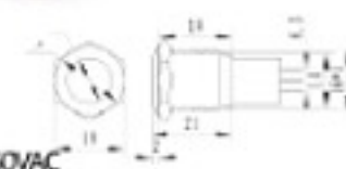
S1601A 16mm不鏽鋼金屬平面環形燈無段開關
