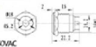
S16002B 16mm不鏽鋼金屬平面有段開關(單刀)
