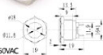
S16013A 16mm不鏽鋼金屬平面環形燈無段開關(焊線式)
