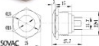
S22002A 22mm不銹鋼金屬平面無段開關
