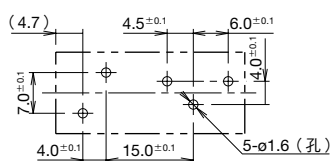
• PCB 加工圖 (BOTTOM VIEW)
