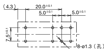
• PCB 加工圖 (BOTTOM VIEW)
