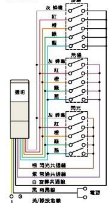
旋轉閃光 蜂鳴型(RS)
