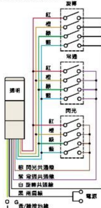
旋轉閃光型(RF)
