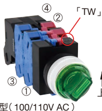
變壓器型(100/110V AC)
