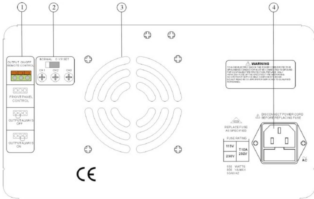
Fig.1.4-1 後面板圖
