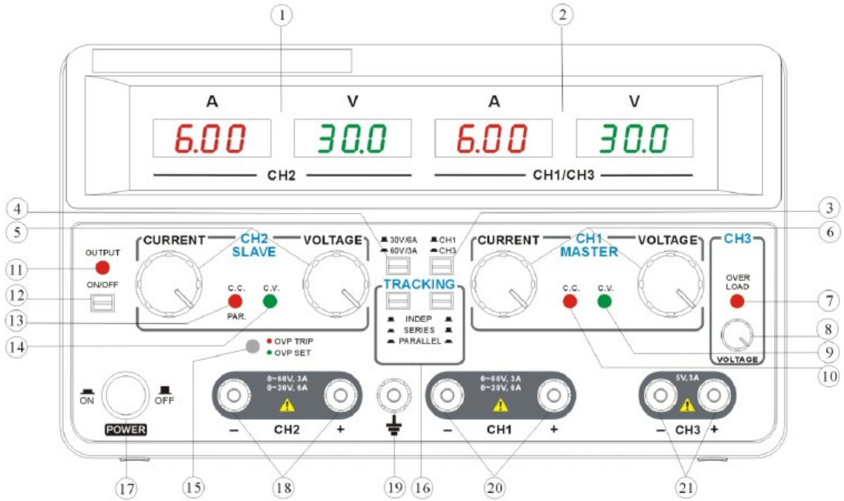
Fig.1.3-1 前面板圖
