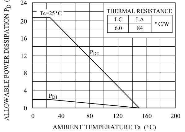
Fig. 11 P_D - T_a (API-Type : TO-220IS)
